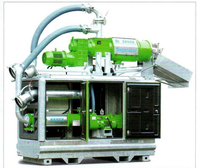
Das „Plug & Play“ Separator-System ist schnell umsetzbar.
